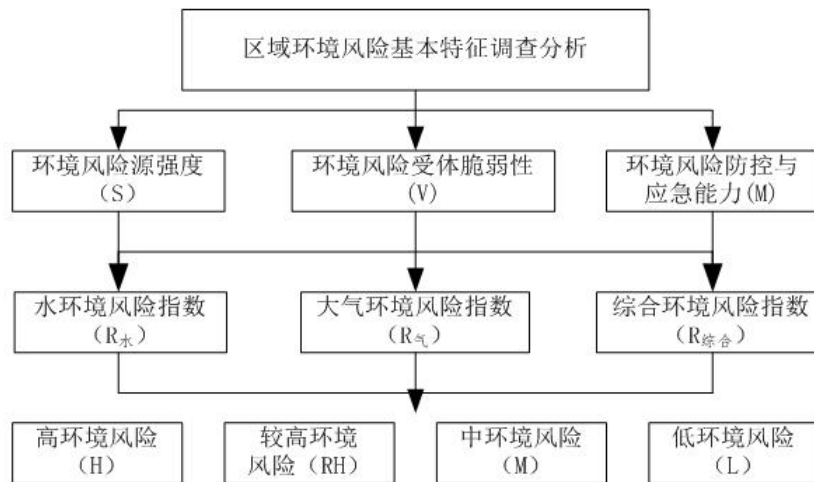
图 2 行政区域突发环境事件风险等级划分程序
